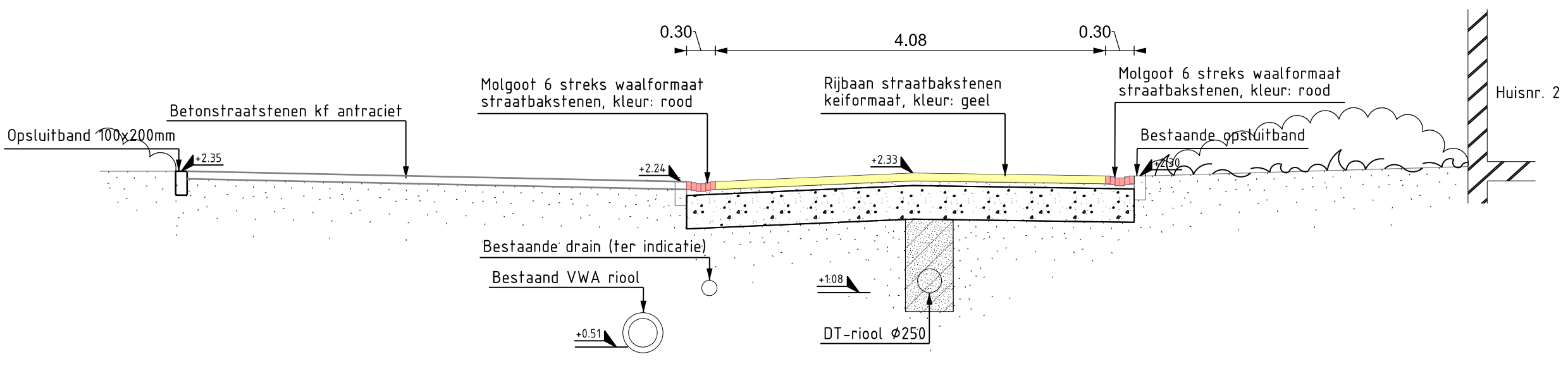
Principe doorsnede C C SCHAAL 1 : 50
