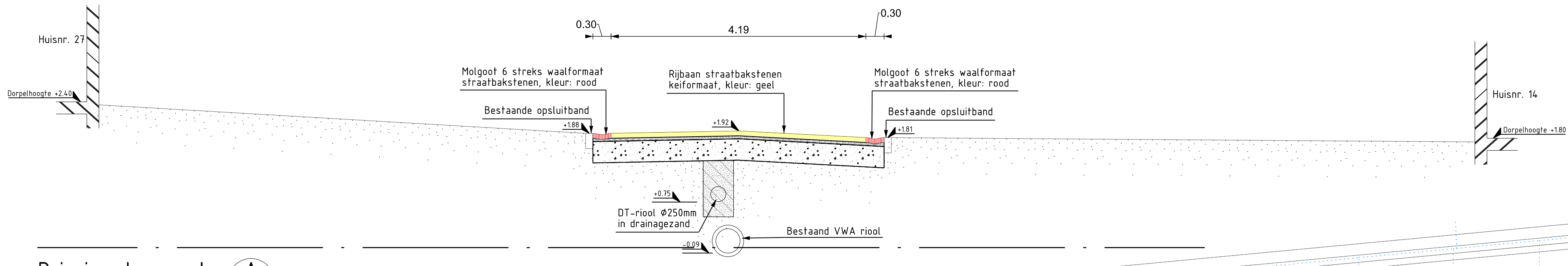
Principe doorsnede A A SCHAAL 1 : 50
