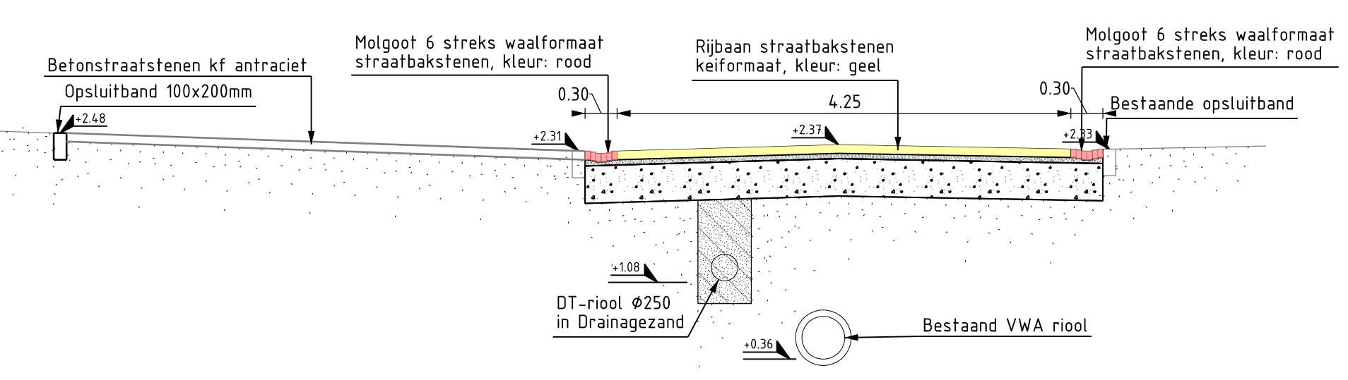
Principe doorsnede B B SCHAAL 1 : 50
